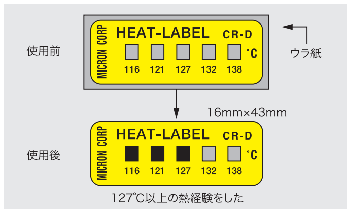
図1. 5点表示ラベル(実物大)
