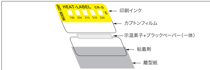
高温レンジ構造図 CR-E~J 6R-166~241 MN全レンジ
