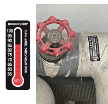
可逆性温度計ラベルSCA
